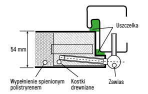
PROFIL SKRZYDŁA
