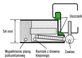
PROFIL SKRZYDŁA
