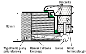
PROFIL SKRZYDŁA
