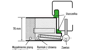
PROFIL SKRZYDŁA
