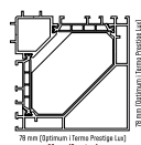
Rysunek techniczny
