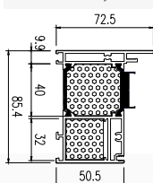
Rysunek techniczny
