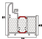
Rysunek techniczny
